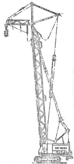
СКГ-40/63: башенно-стреловое исполнение
